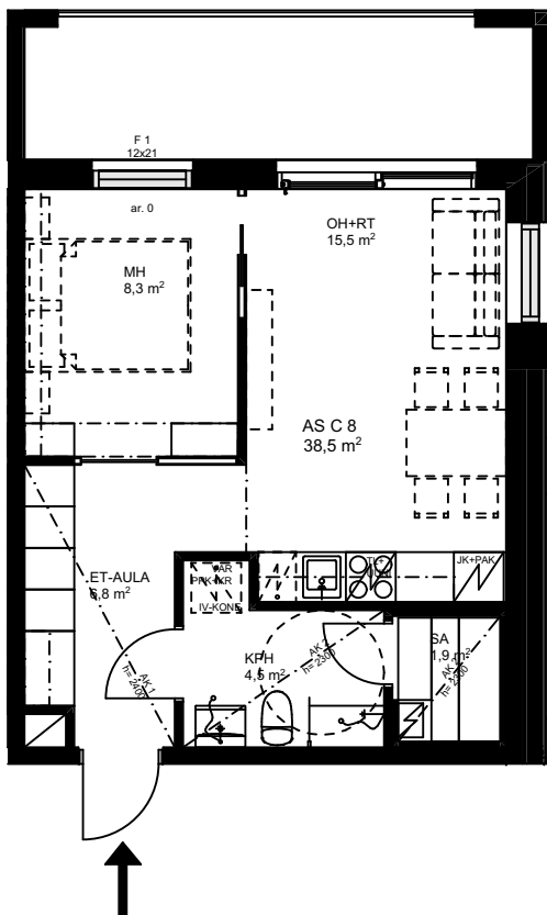
POHJAPIIRUSTUS 1:100
